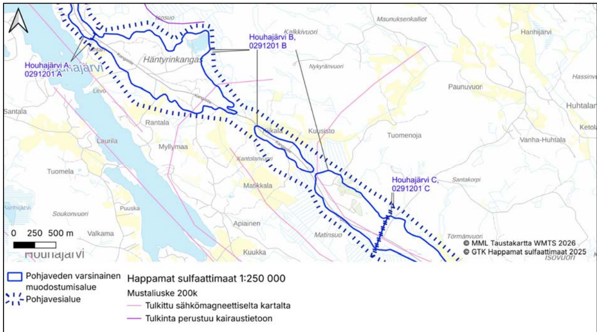
Kuva 15. Mustaliuske-esiintymät pohjavesialueella Houhajarvi B.
