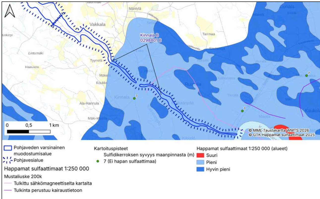
Kuva 6. Happamat sulfaattimaat ja mustaliuske-esiintymät pohjavesialueella Kinnala B.
