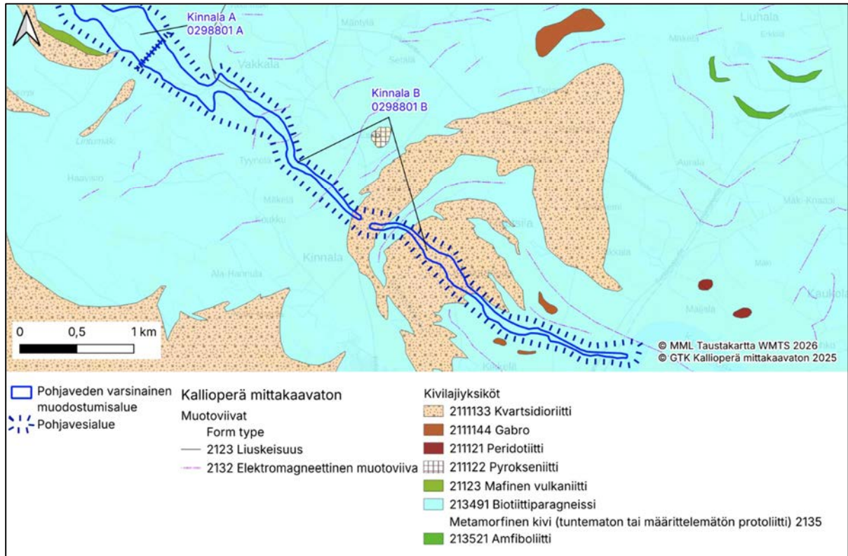
Kuva 5. Kallioperä pohjavesialueella Kinnala B.
