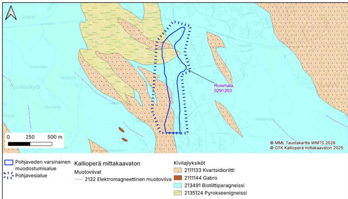
Kuva 19. Kallioperä pohjavesialueella Roismala.
