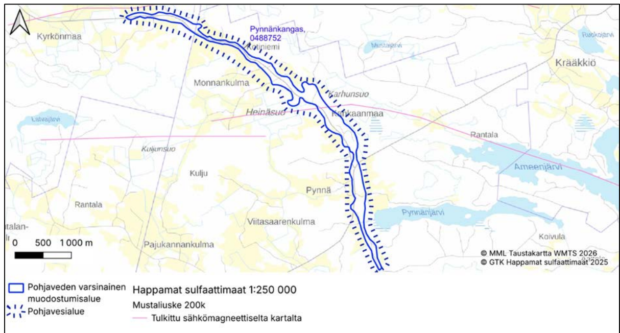
Kuva 24. Mustaliuske-esiintymät pohjavesialueella Pynnänkangas.
