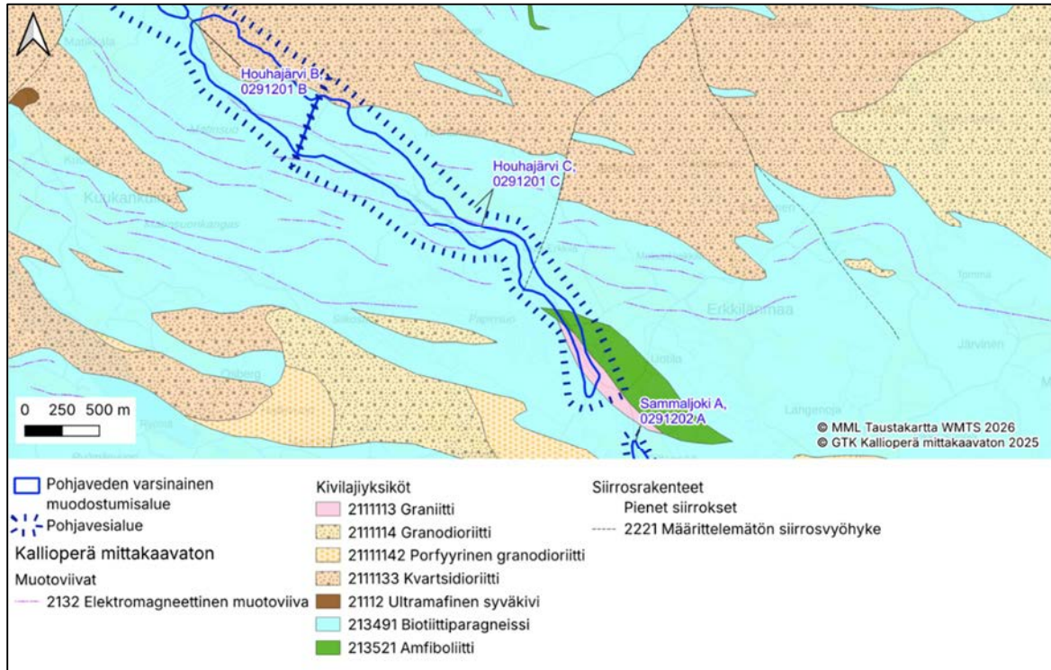
Kuva 16. Kallioperä pohjavesialueella Houhajarvi C.
