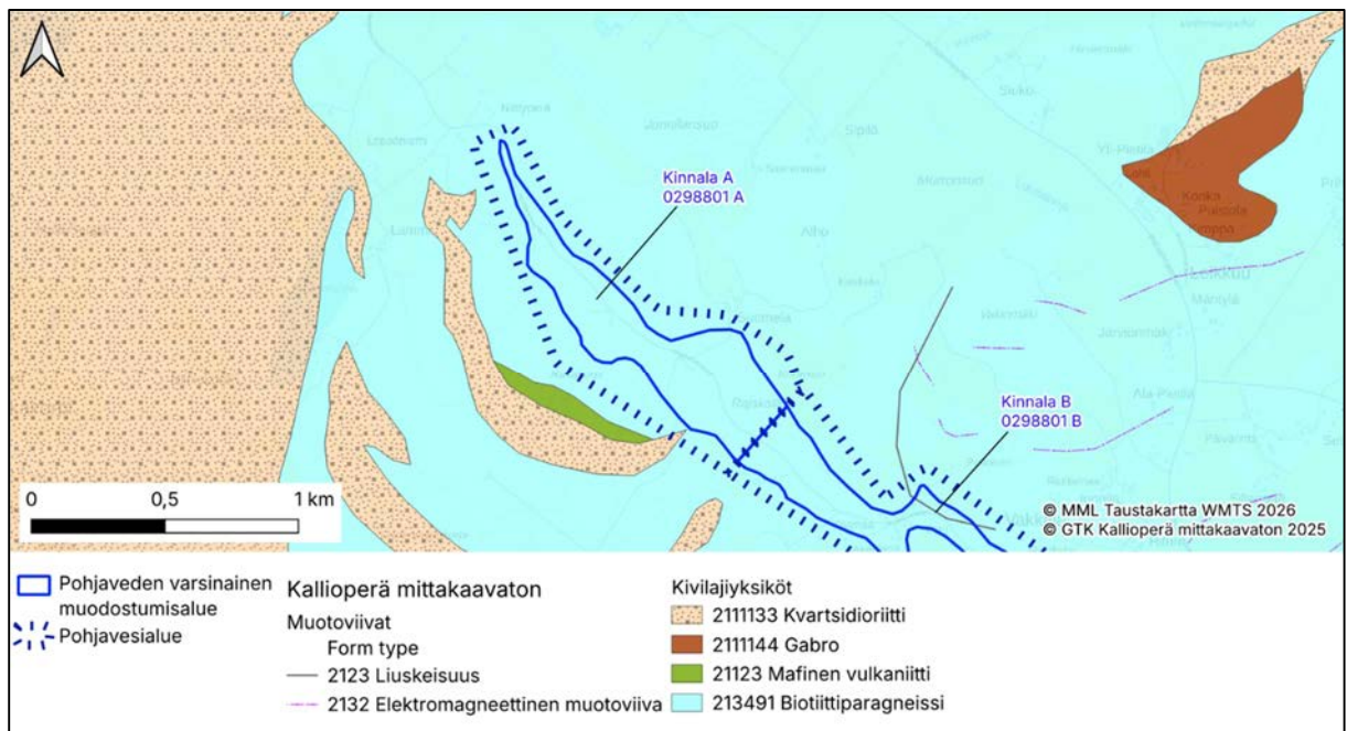
Kuva 4. Kallioperä pohjavesialueella Kinnala A.
