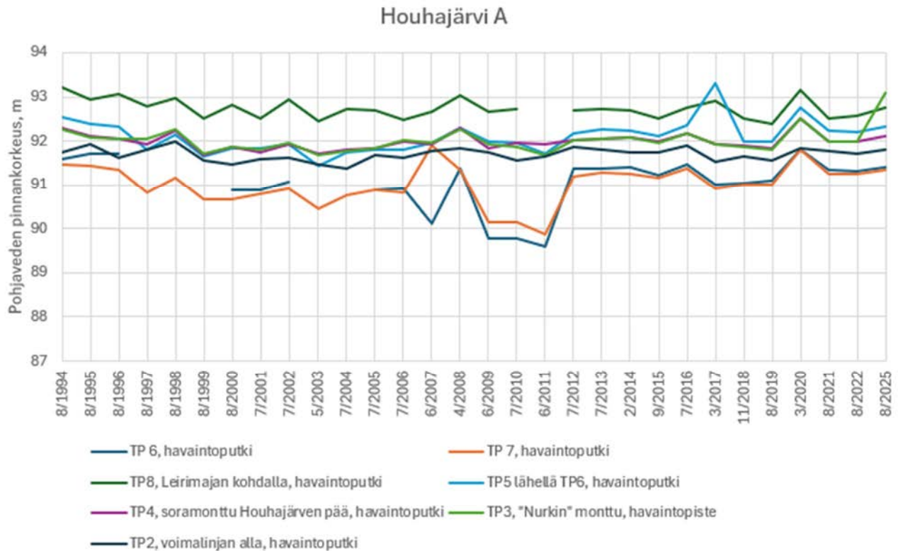
Kuva 13. Pohjaveden pintojen seuranta ajanjaksolla 1994–2025. Vuosilta 2023 ja 2024 ei ole mittaustuloksia.
