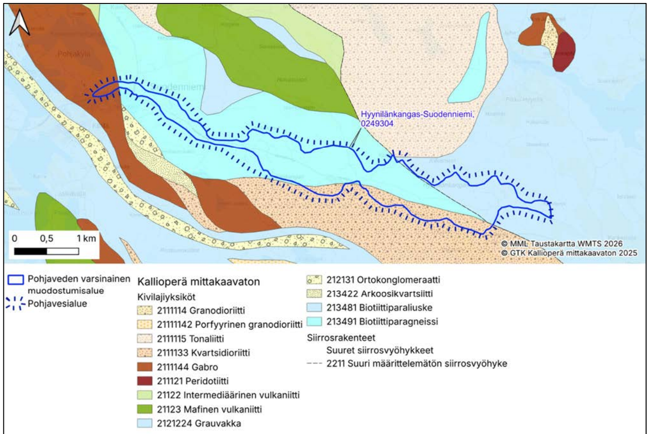
Kuva 1. Kallioperä pohjavesialueella Hyynilänkangas-Suodenniemi.
