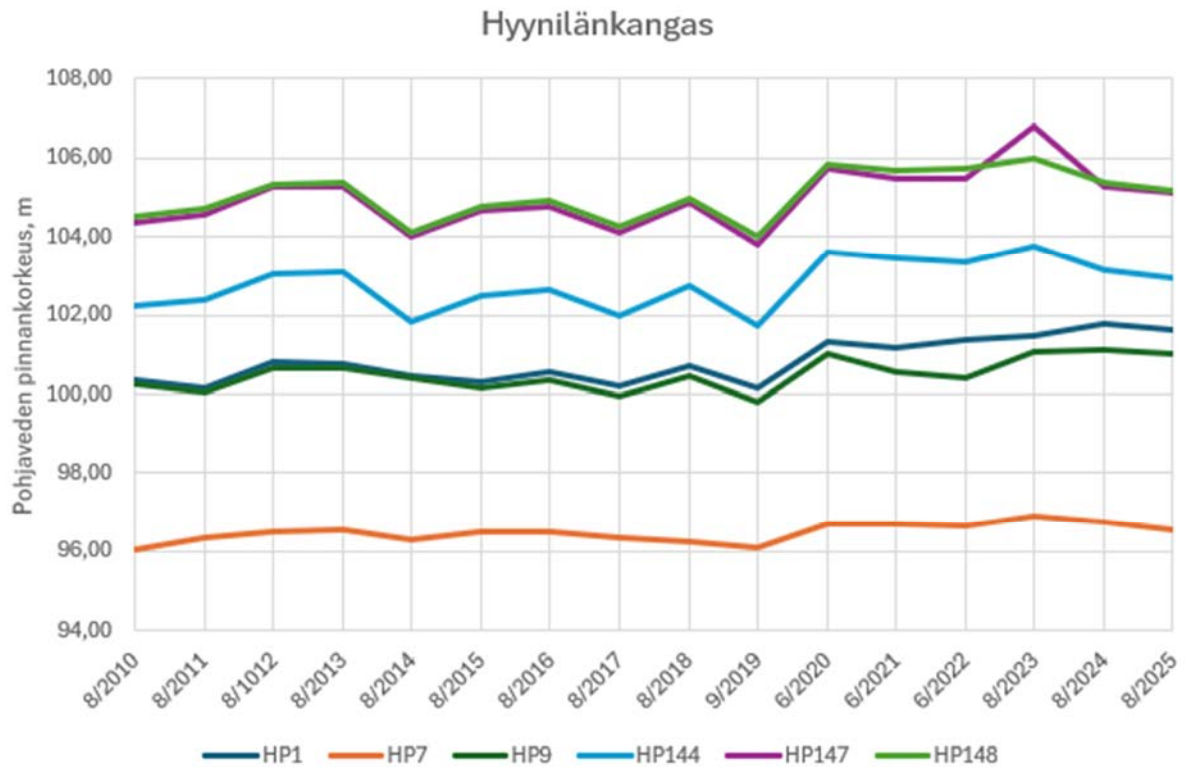
Kuva 3. Pohjaveden pintojen seuranta ajanjaksolla 2010–2025.
