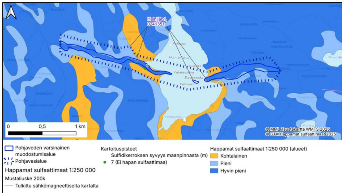
Kuva 22. Hapamat sulfaattimaat pohjavesialueella Heinijärvi.
