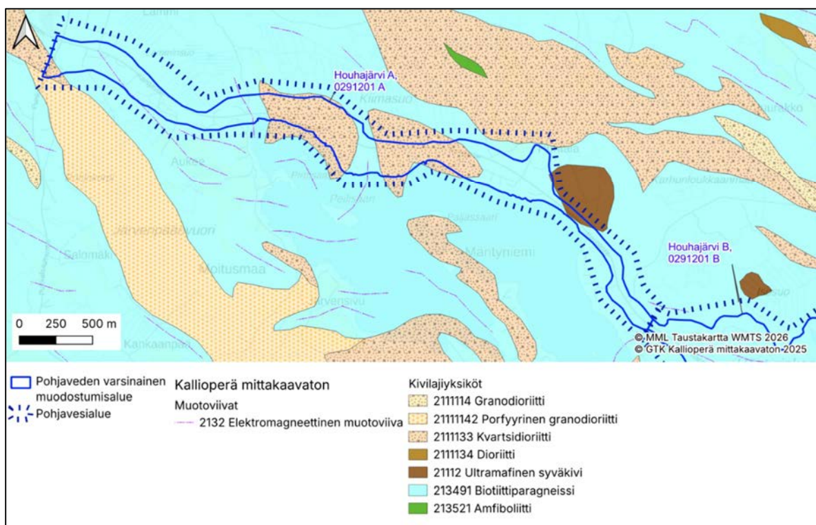
Kuva 11. Kallioperä pohjavesialueella Houhajärvi A.
