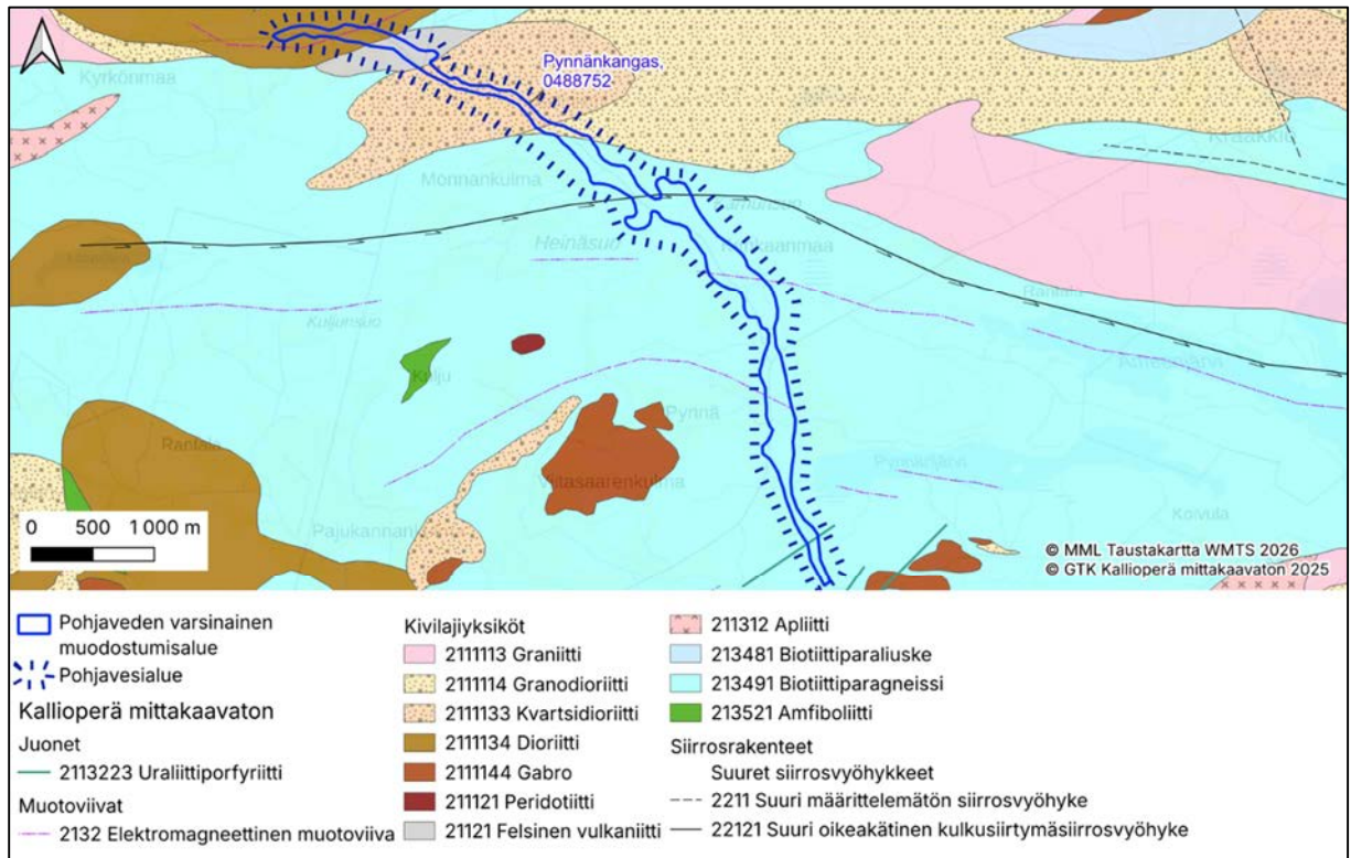
Kuva 23. Kallioperä pohjavesialueella Pynnänkangas.
