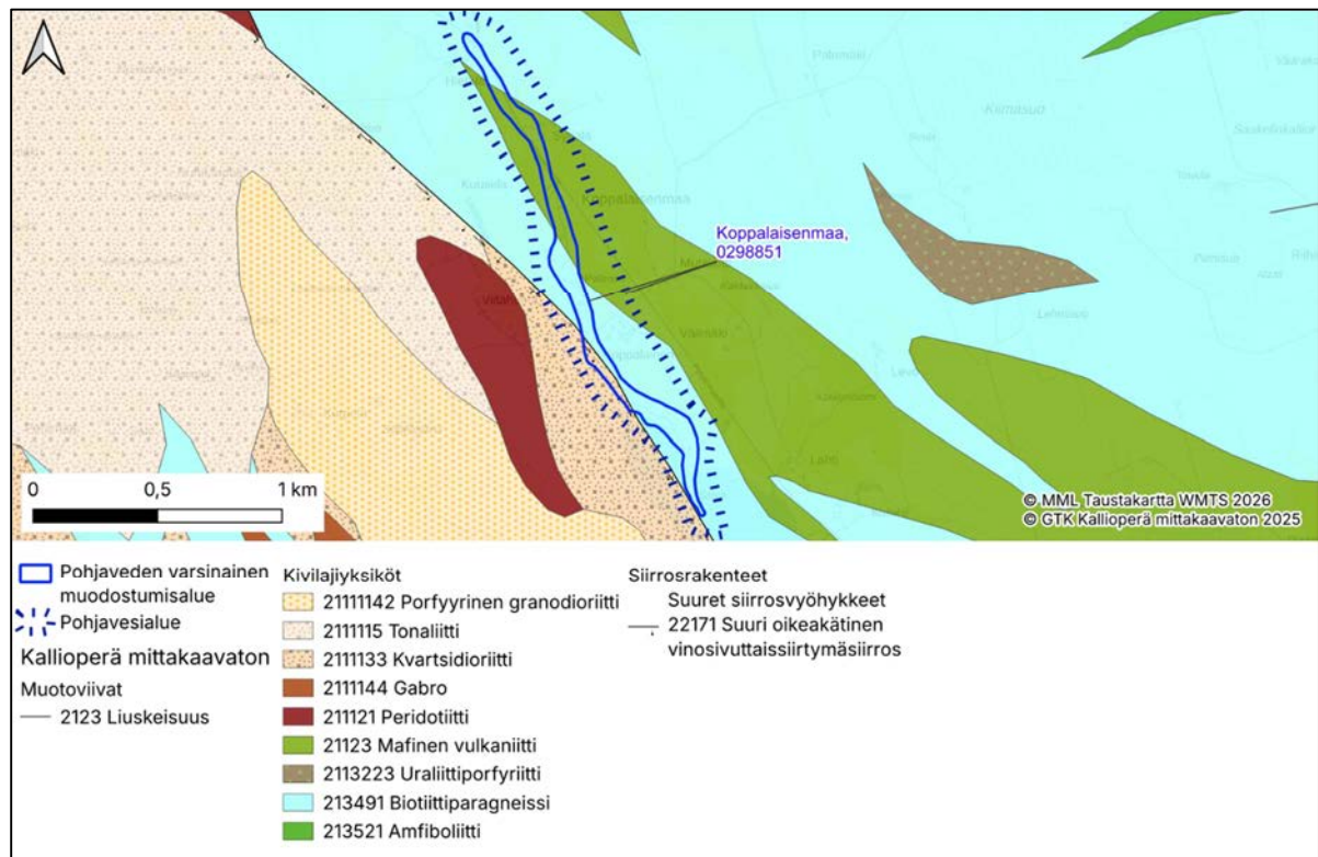
Kuva 8. Kallioperä pohjavesialueella Koppalaisenmaa.
