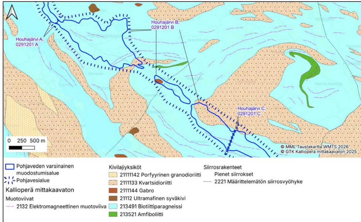
Kuva 14. Kallioperä pohjavesialueella Houhajarvi B.
