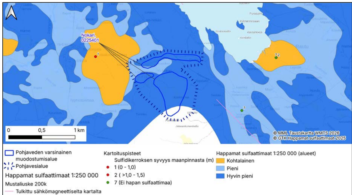
Kuva 10. Happamat sulfaattimaat pohjavesialueella Nokari.
