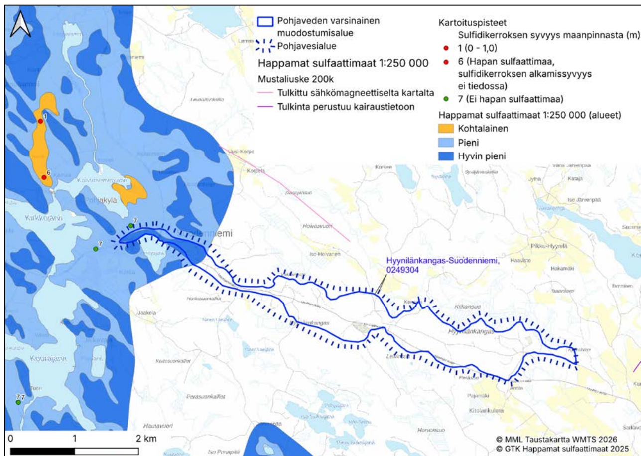
Kuva 2. Happamat sulfaattimaat ja mustaliuske-esiintymät Hyynilänkangas-Suodenniemi-pohjavesialueella ja sen läheisyydessä.
