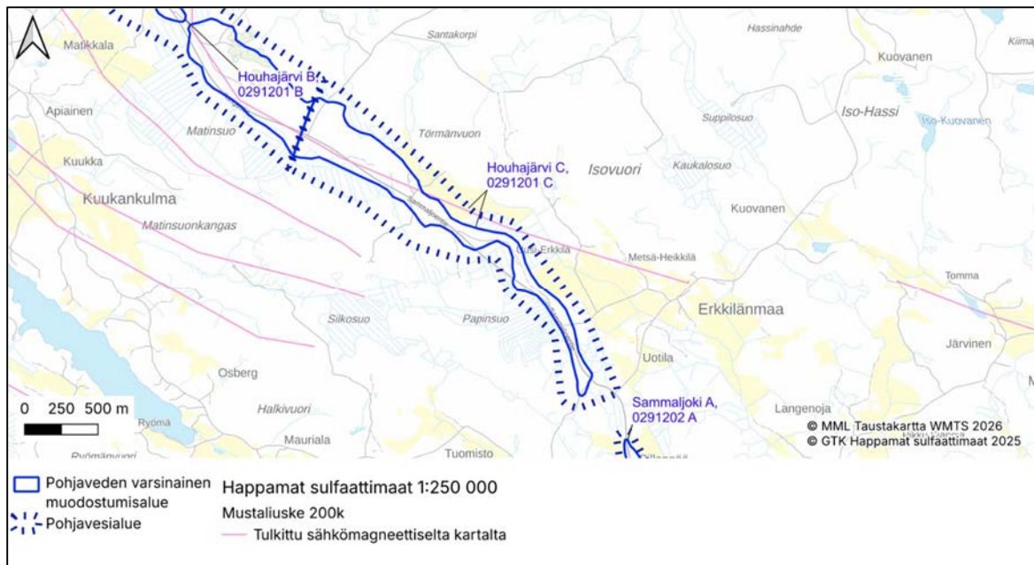
Kuva 17. Mustaliuske-esiintymät pohjavesialueella Houhajarvi C.
