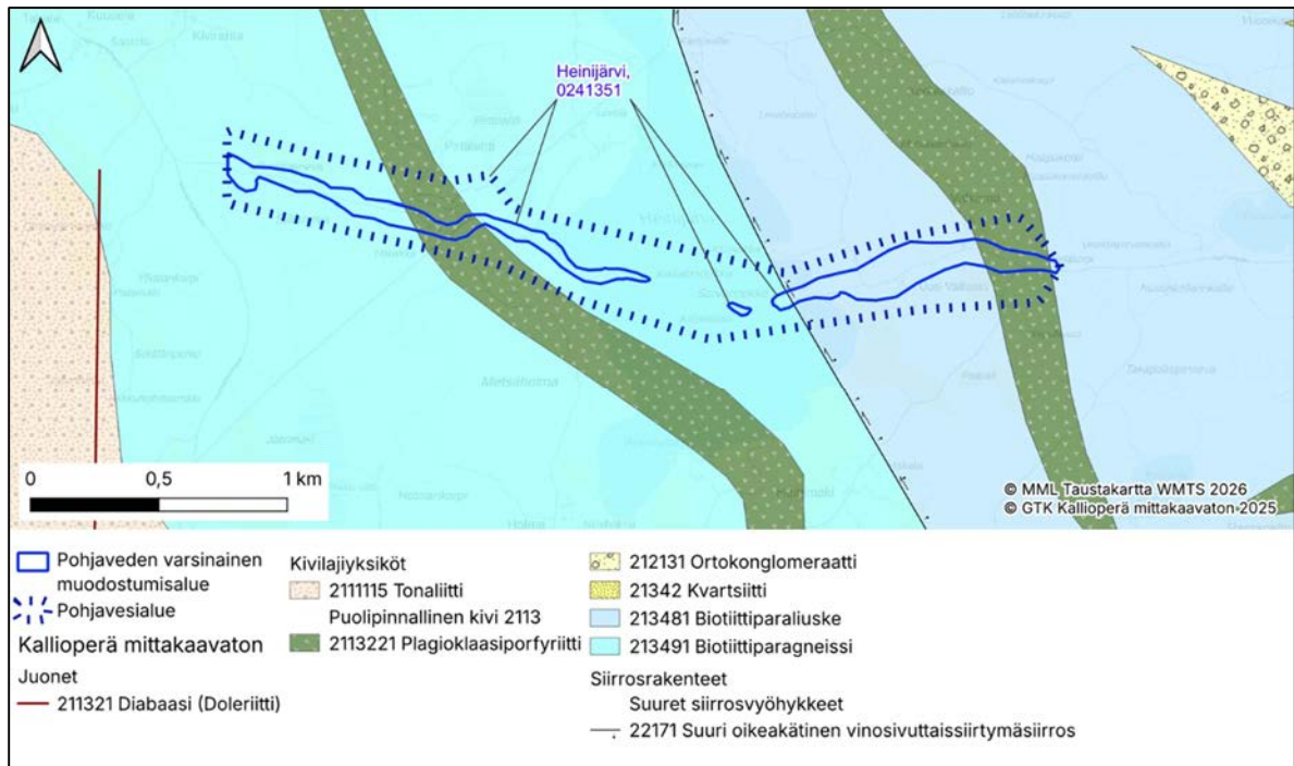
Kuva 21. Kallioperä pohjavesialueella Heinijärvi.
