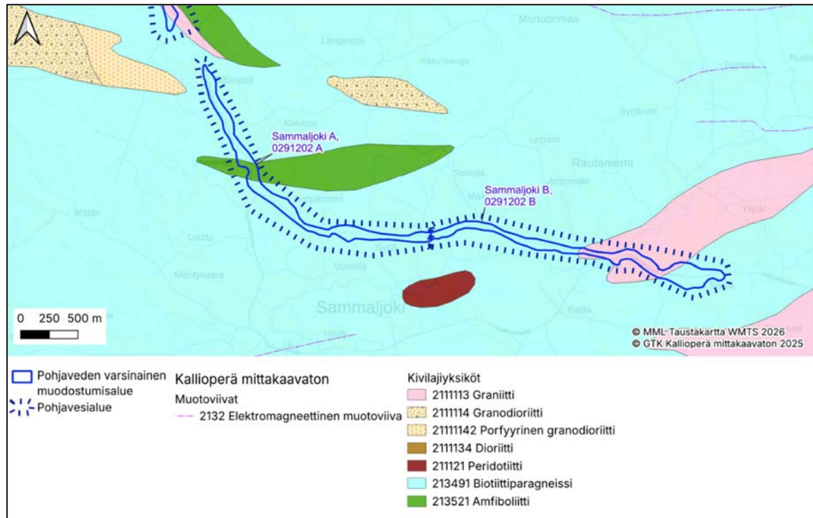
Kuva 18. Kallioperä pohjavesialueilla Sammaljoki A ja Sammaljoki B.
