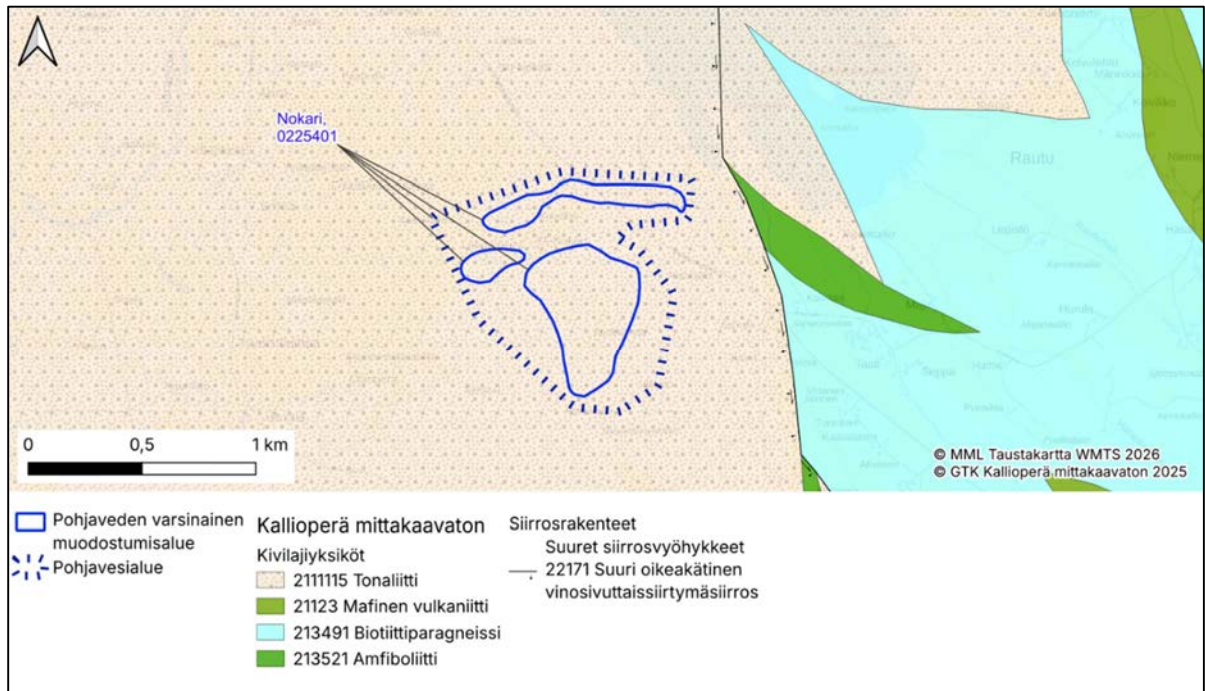
Kuva 9. Kalliojärvi pohjavesialueella Nokari.
