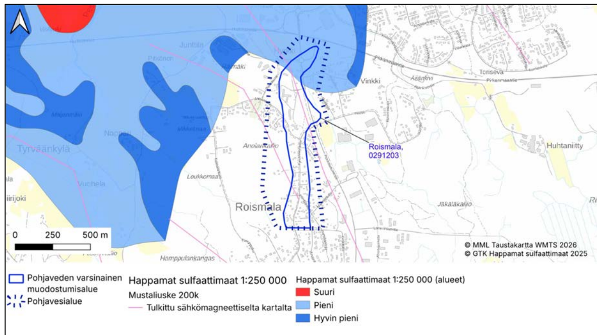
Kuva 20. Happamat sulfaattimaat ja mustaliuske-esiintymät pohjavesialueella Roismala.
